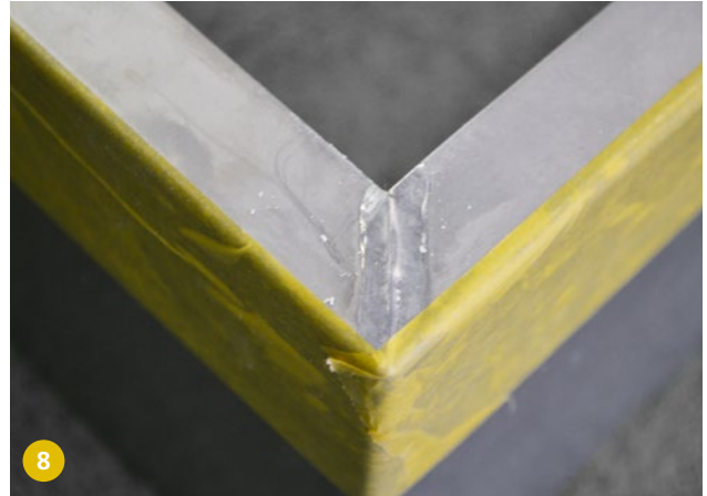
8 Gehrungen und Anschlussboden sind dicht auszuführen.
